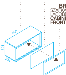
BR 91 SZAFKA Z FRONTEM Z PŁYTY LAMINOWANEJ CABINET WITH LAMINATED BOARD FRONT
