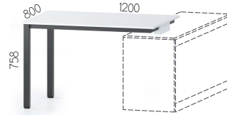
WGBN2/8
