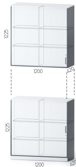
WGSAZ4
