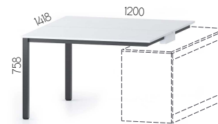
WGBN12
