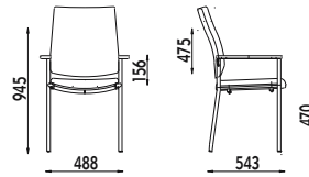
ZEN 212
