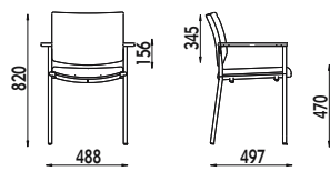
ZEN ARM 112
