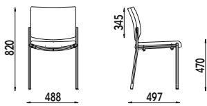
ZEN 102
